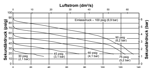
3/8-ZOLL-FILTER/REGLER BAUREIHE 1500
