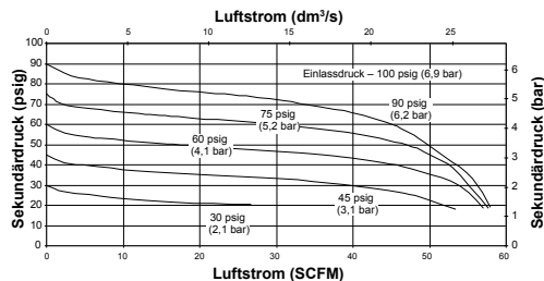
1/4-ZOLL-FILTER/REGLER BAUREIHE 1000
