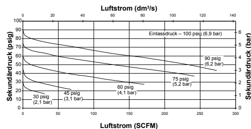
3/4-ZOLL-F-R-L-KOMBINATION BAUREIHE 3000
